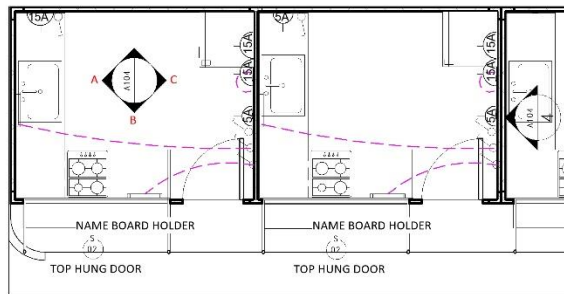
2. ELECTRICAL PLAN 1 : 50
