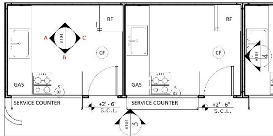
1. PROTOTYPE PLAN 1 : 50
